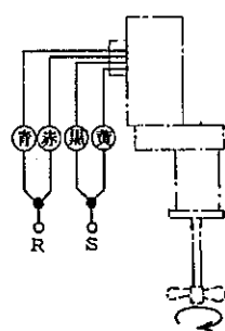
■単相 100V 単相モーター結線
