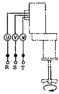
■3相 200V (400V) 3相モーター結線
