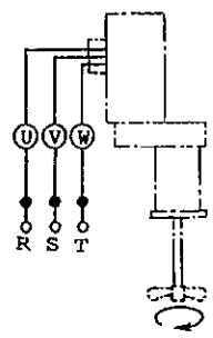
■ 3相 200V (400V) 3相モーター結線
