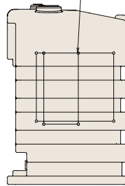
4-M4×2操作盤取付インサート
